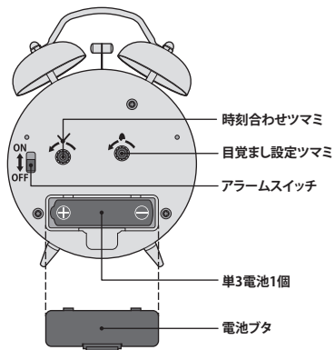
本体後面
